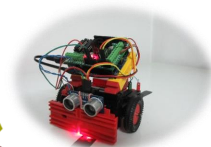
Fotografija robota v akciji
